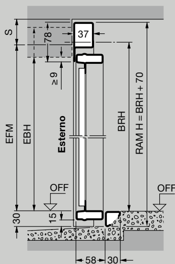
Sezione verticale Montaggio oltre luce
