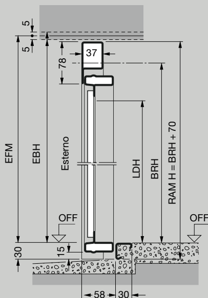
Sezione verticale Montaggio oltre luce
